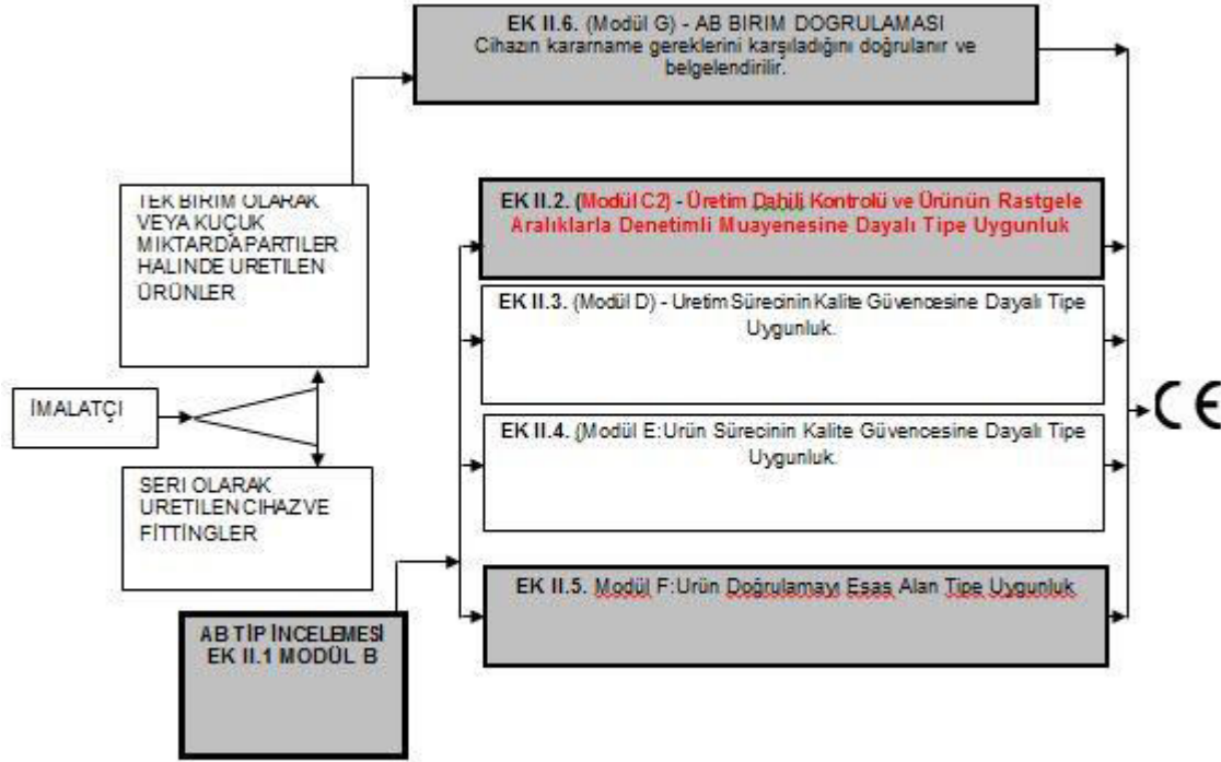
Şekil 2 Uygunluk değerlendirme süreçleri (firmanın uyguladığı modüller gri ile belirtilmiştir)
